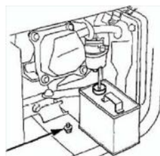
ДРЕНАЖНЫЙ БОЛТ
