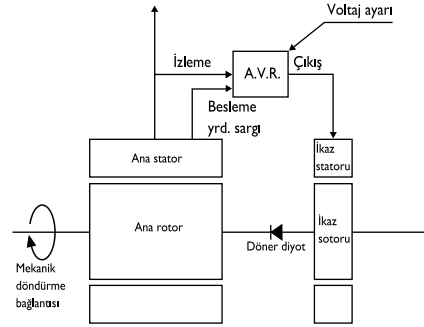
Şekil 11.1. Alternatör çalışması blok şeması
